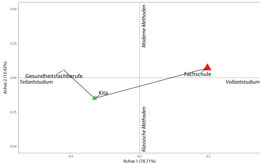
Abb. 8: Raum der Interessenslagen – Strukturierender Faktor: Berufsgruppen
