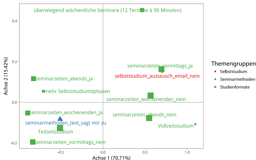
Abb. 2: Raum der Interessenslagen – Punktwolke der Kategorie (Achse 1)
