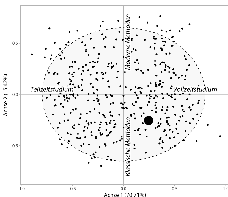
Abb. 4: Raum der Interessenslagen – Punktwolke der Individuen
