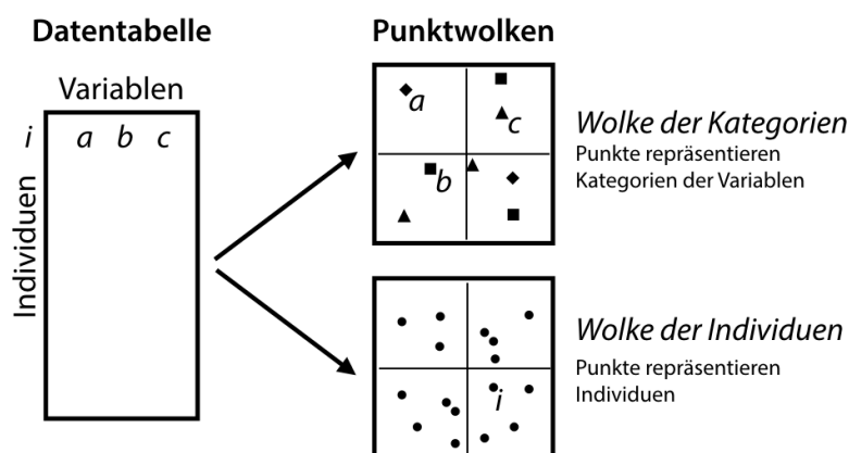
Abb. 1: Datensatz und die beiden resultierenden Punktwolken (in Anlehnung an Le Roux & Rouanet 2010, S. 2)
